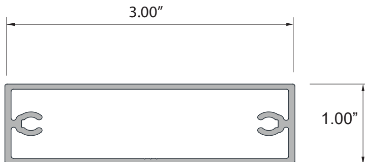
1" x 3" Batten
