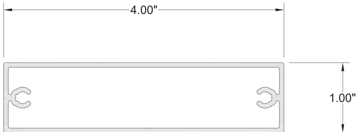
1" x 4" BATTEN
