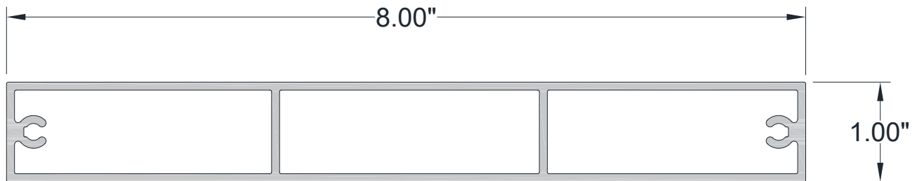
1" x 8" BATTEN
