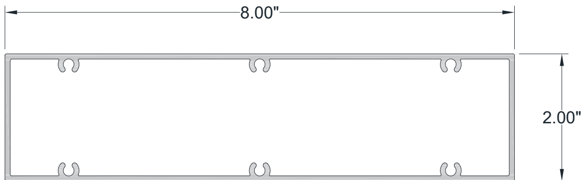
2" x 8" BATTEN
