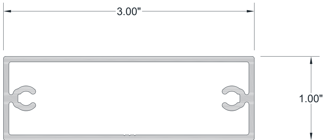
1" x 3" BATTEN
