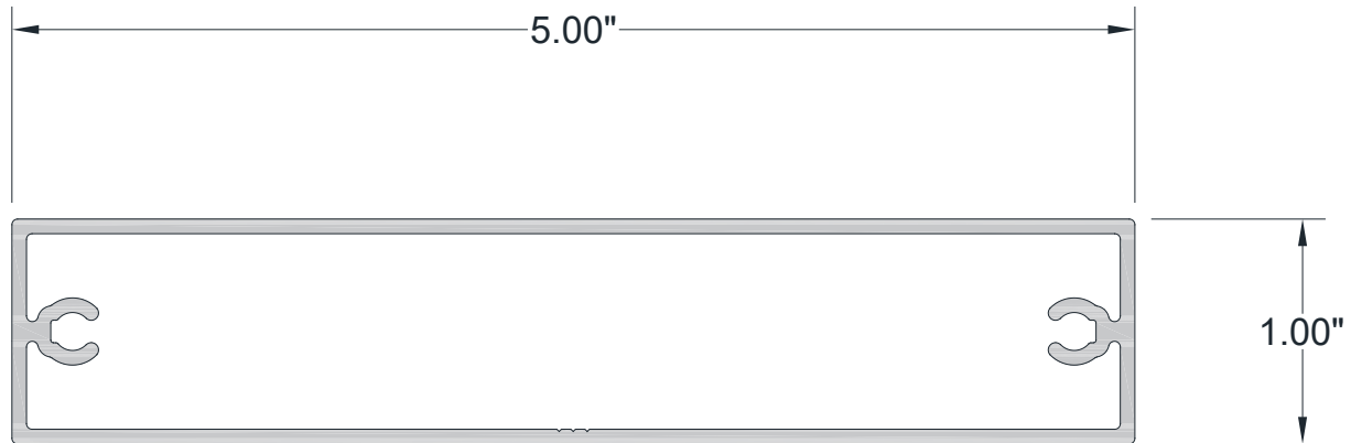
1" x 5" BATTEN
