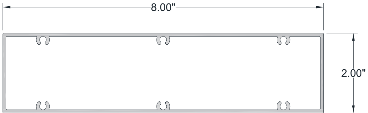
2" x 8" BATTEN
