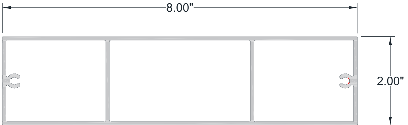
2" x 8" BATTEN
