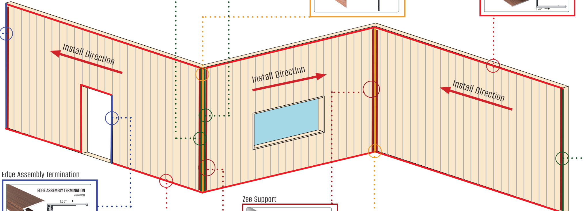
J-Starter
