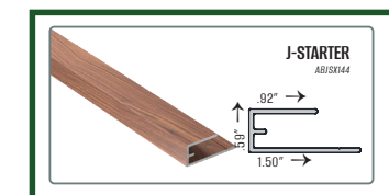
J-Starter
