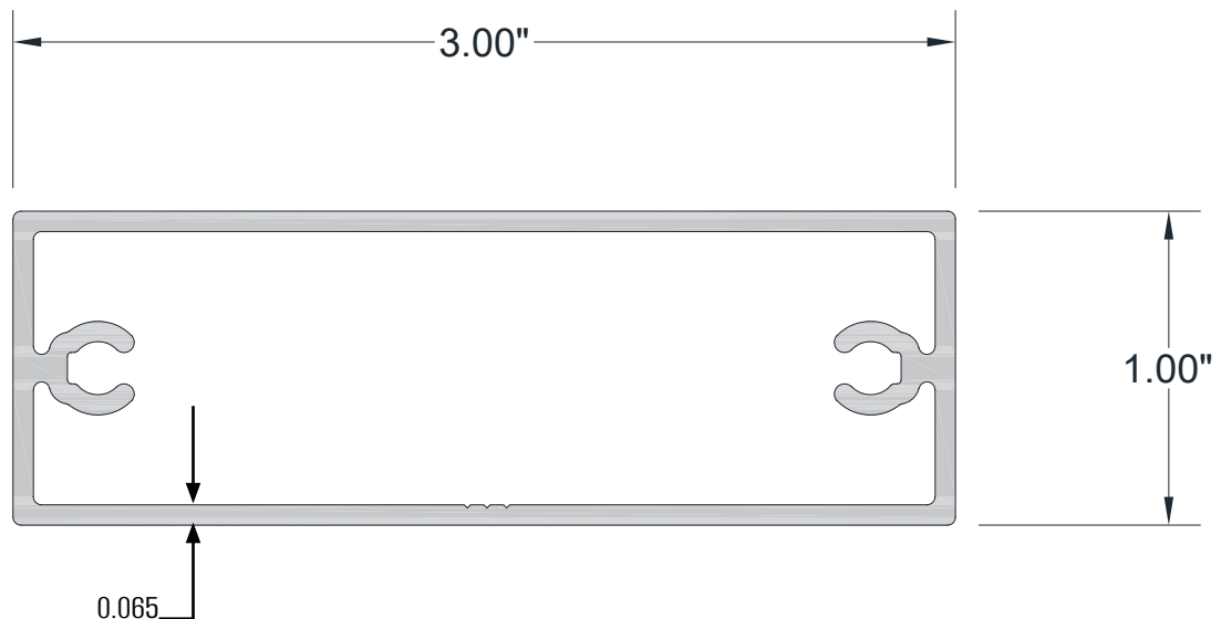
1" x 3" BATTEN
