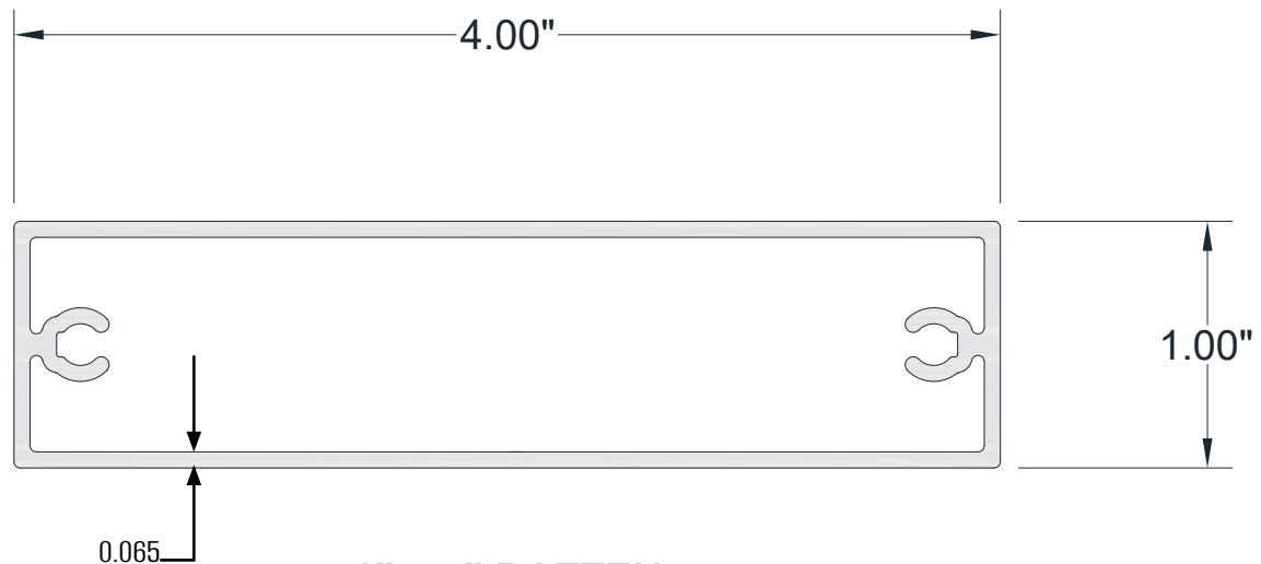
1" x 4" BATTEN
